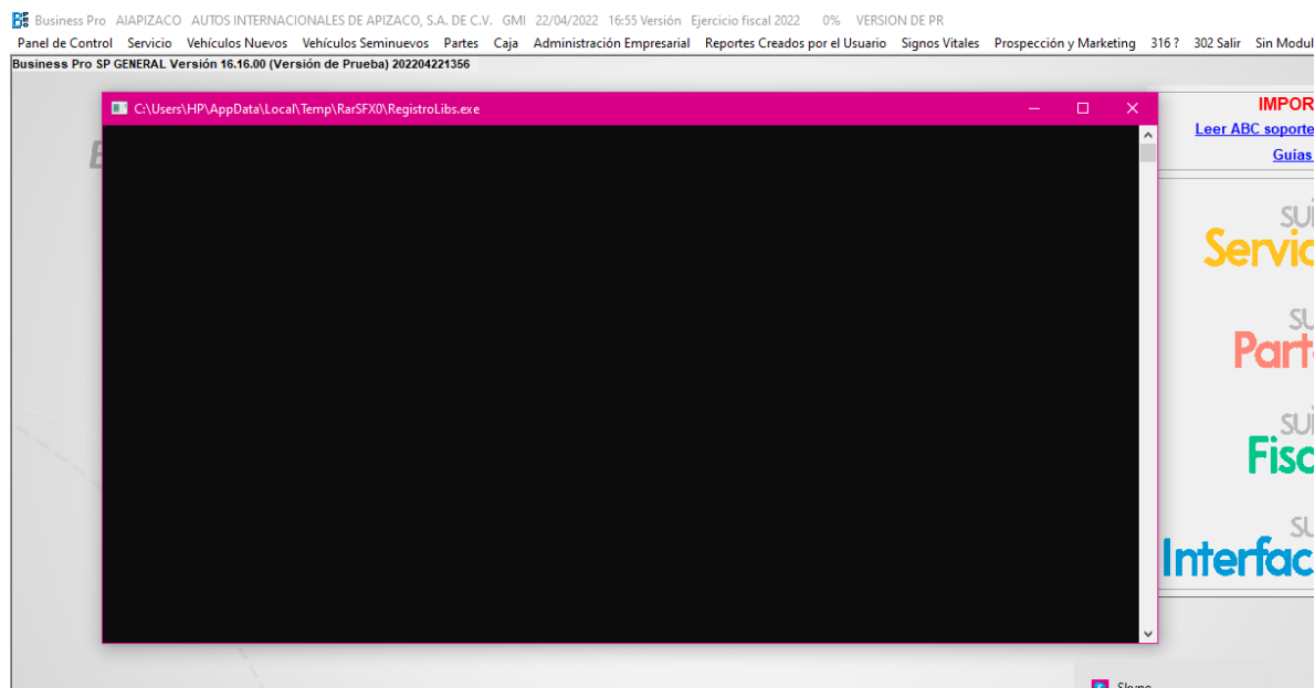
Fig. 8 Ventana MS-DOS
